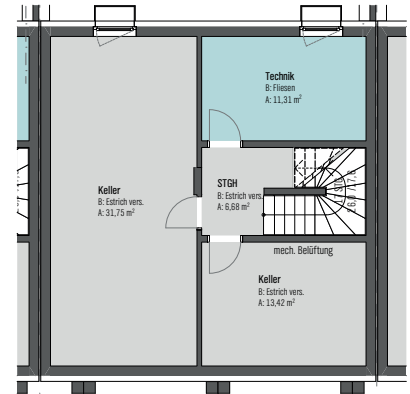
KELLERGESCHOSS ohne Masstab
